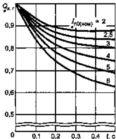
Рисунок 12 - Кривые для определения Q синхронных генераторов с тиристорной независимой системой возбуждения
