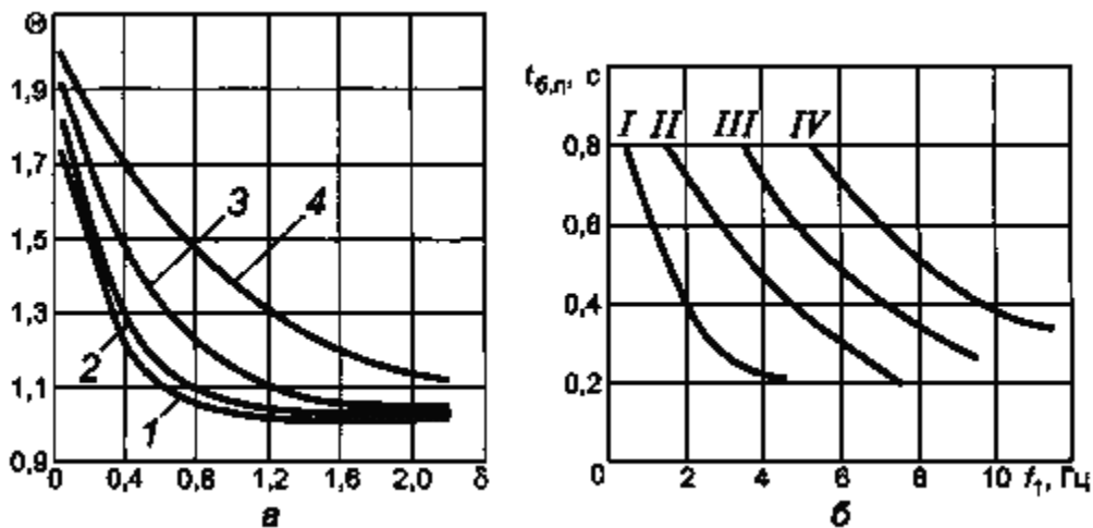
Рисунок Б.1 - Определение коэффициента превышения напряжения и нагрузки \Theta в зависимости от \delta , t_{б.п} и f_1
