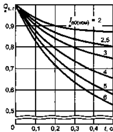
Рисунок 13 - Кривые для определения Q синхронных генераторов с тиристорной системой самовозбуждения
