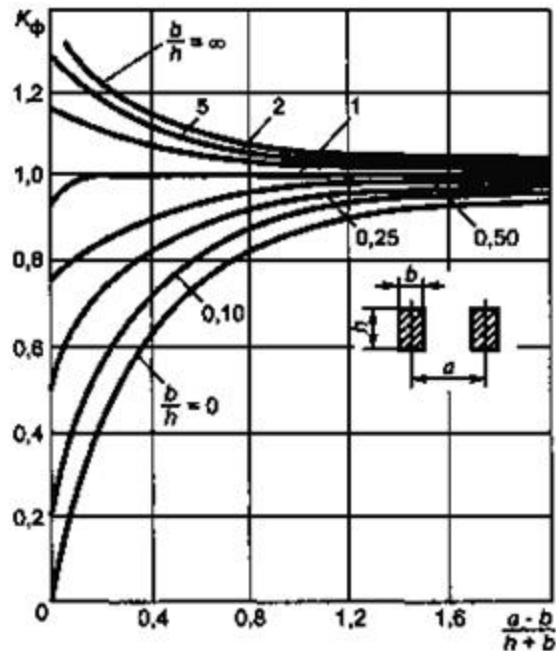
Рисунок 1 - Диаграмма для определения коэффициента формы проводников прямоугольного сечения
