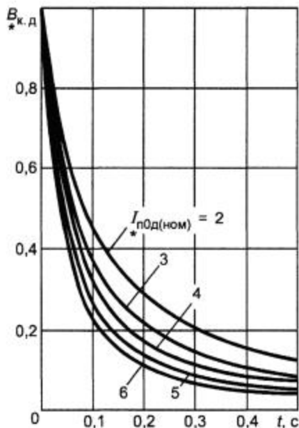
Рисунок 17 - Кривые для определения
