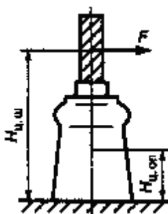
Рисунок 8 - К расчету приведенной массы опоры
