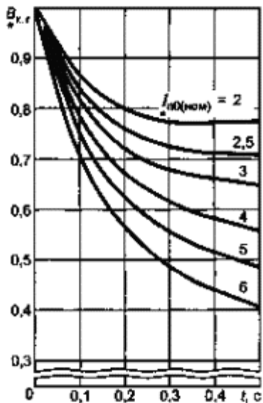
Рисунок 9 - Кривые для определения t_{к.з.} от синхронных генераторов с тиристорной независимой системой возбуждения
