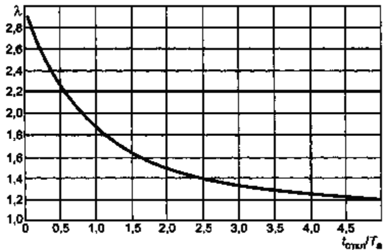
Рисунок В.1 - Зависимость коэффициента \lambda от t_{\text{откл}}/T_a
