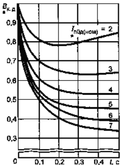
Рисунок 15 - Кривые для определения
