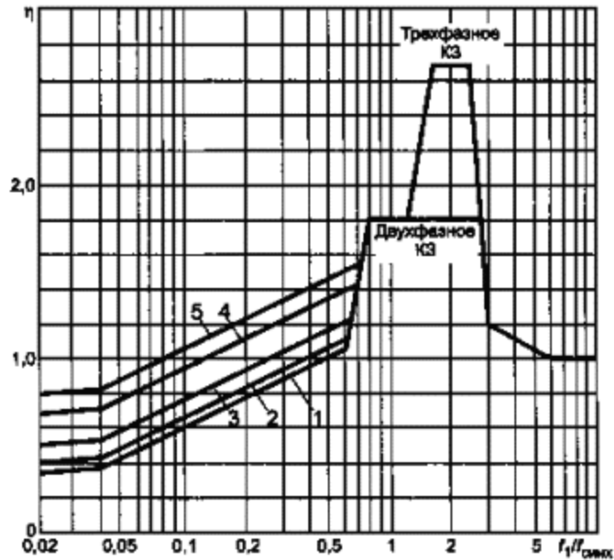
Рисунок 5 - Зависимость коэффициента динамической нагрузки для изоляторов и шин от частоты собственных колебаний шины при различных ударных коэффициентах \chi : 1 - \chi \geq 1,6 ; 2 - \chi = 1,4 ; 3 - \chi = 1,25 ; 4 - \chi = 1,1 ; 5 - \chi = 1,0
