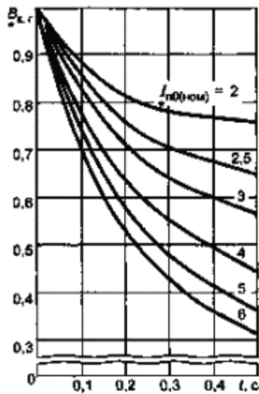
Рисунок 10 - Кривые для определения t_{к.з.} от синхронных генераторов с тиристорной системой самовозбуждения
