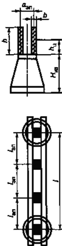
Рисунок 4 - Двухполосная шина
