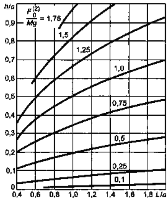
Рисунок В.3 - Характеристики h/a = f(L/a) при двухфазном КЗ
